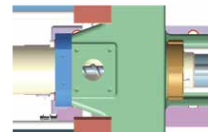
■ 自動鎖固螺桿逆流圈設計（選配項目）。 Auto-lock check ring design. (optional accessories)
