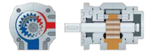
德國高效率內接齒輪泵剖面圖
